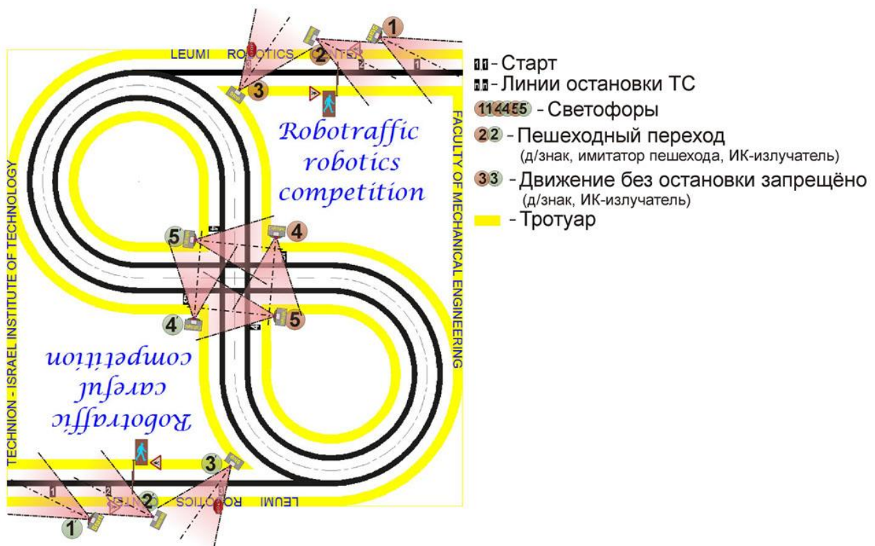
Рис. Оснастка поля категории А - Модель "городского уличного движения" (РобоТраффик - 2024)
